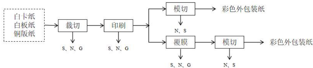
图 3-1 生产工艺流程及产污节点图（G—废气；S—固体废弃物；N—噪声）
